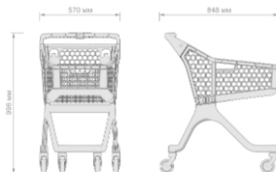
Габариты изделия
